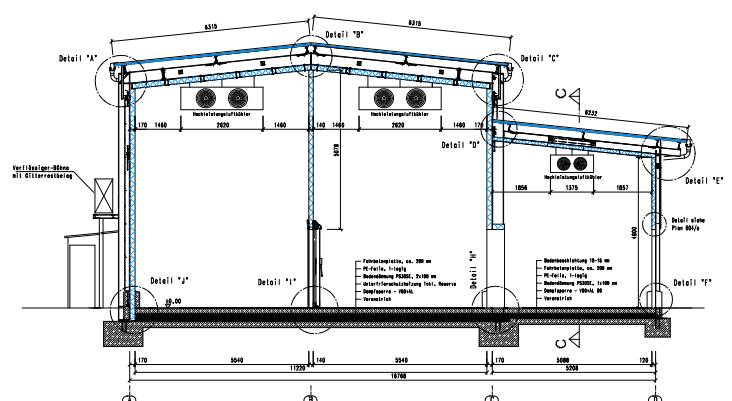
Schnitt A-A
