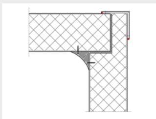
Vorgefertigtes, gerundetes Inneneckprofil
