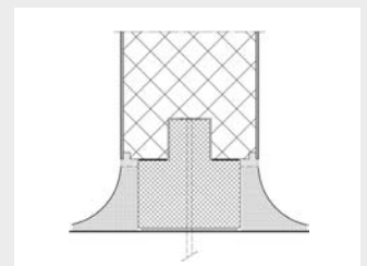
Wandbündiger Hohlkehl-Bodenanschluss
