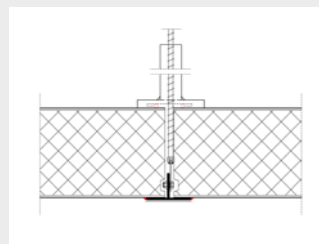
Kältebrückenfreie, hygienisch einwandfreie Deckenabhangung
